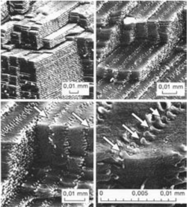
Bild 3: Mikroskopische Struktur der Augenlinse. Die vier unterschiedlich starken Vergrößerungen mit Hilfe des Rasterelektronenmikroskops zeigen die präzise geordnete Schichtenstruktur. Die Länge eines hundertstel Millimeters ist jeweils maßstäblich gezeichnet. Durch einzigartig beschaffene Kugelgelenke (durch Pfeile in den beiden unteren Vergrößerungen markiert) sind die Proteinlagen miteinander zu einem elastischen Verbund vernetzt, sodass unterschiedliche Brennweiten durch Formveränderungen der Linse ermöglicht werden.
